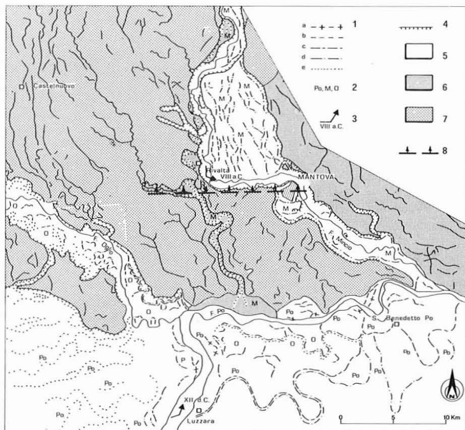
FIG. 9 - Schizzo geomorfologico dell'area di Mantova (da PANIZZA & alii , 1988 a, modificato): 1) Paleovalve a) et  moderna, b) et  basso medioevale, c) et  alto medioevale, d) et  romana e a luoghi del ferro, e) et  del bronzo; 2) Sigle dei paleovalvei: Po = Po, M = Mincio, O = Oglio; 3) Principali deviazioni fluviali con indicazione dell'et ; 4) Scarpa; 5) Depositi alluvionali abbandonati dai corsi d'acqua o dai paleovalvei che li attraversano e quindi ad essi coevi; 6) Depositi alluvionali sub-boreali (recenti nelle vicinanze degli alvei attuali) del Mincio, Tartaro ed Adige con paleovalvei coevi; 7) Depositi fluvio-glaciali di pertinenza gardesana con tracce di canali proglaciali; 8) Asse di deformazione ritenuto attivo (freccie verso la zona pi  abbassata).
