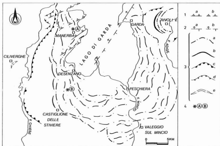
FIG. 10 - Schizzo geomorfologico del settore meridionale del L. di Garda: 1) Sovrascorrimiento ritenuto attivo a) in affioramento, b) coperto (triangoli sulla parte sovrascorsa); 2) Faglia inversa ritenuta attiva a) in affioramento, b) coperta (tratti verso la zona abbassata, frecce secondo l'immersione); 3) Morene frontali (da CREMASCHI, 1987), a) fase di Solferino (Pleistocene sup.), b) fase di Sedena (Pleistocene medio), c) fase di Carpendolo (Pleistocene medio), d) fase di M. Faita (Pleistocene medio), e) fase di Ciliverghe (Pleistocene inf.); 4) Ubicazione degli affioramenti di fig. 11 e 12.
