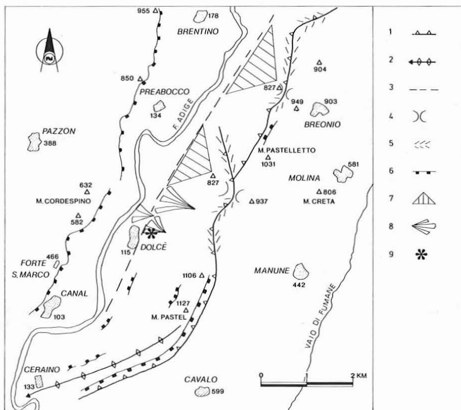
FIG. 13 - Schizzo morfoneotettonico dell'area di Dolcè: 1) Faglia inversa, con debole sovrascorrimento, ritenuta attiva (triangoli verso la zona sovrascorsa); 2) asse di anticlinale ritenuta attiva (freccia secondo l'immersione assiale); 3) Lineamento qualificato; 4) Sella; 5) Vallecola rettilinea; 6) Scarpata; 7) Faccetta triangolare; 8) Conoide alluvionale; 9) Ubicazione della cava descritta.
